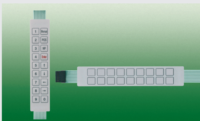
Folientastatur T18.10 und T18.11 , 18 Tasten, mit Druckpunkt, Rückseite mit Klebeschicht
