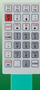
Folientastatur T28.11 , 28 Tasten mit Druckpunkt, Rückseite mit Klebeschicht
